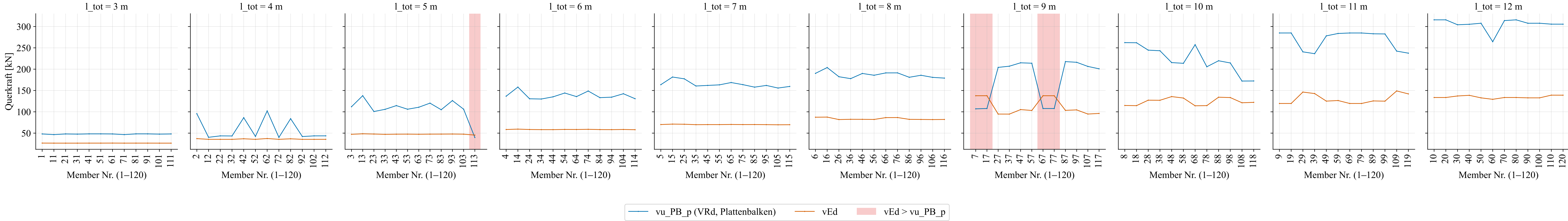
Querkraftwiderstand v_{u\_PB\_p} (VRd, Plattenbalken) vs. Bemessungsquerkraft v_{Ed} je Member, kategorisiert nach Spannweite (Members_rc_rib_simple_massiv_bvar)
